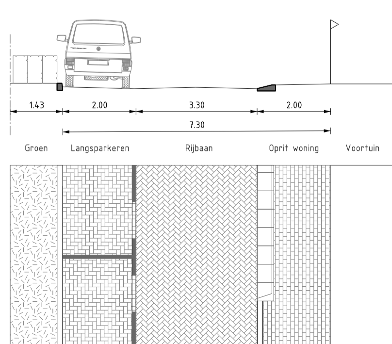
PROFIEL 59 SCHAAL 1 : 100 VO-03 Balistraat
