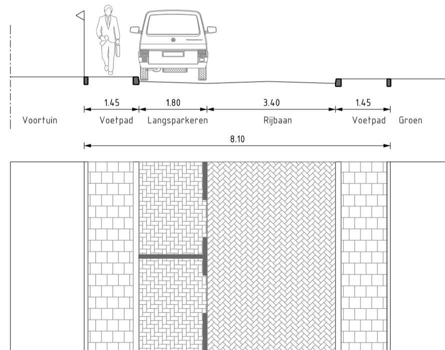
PROFIEL 55 SCHAAL 1 : 100 VO-03 Madoerastraat
