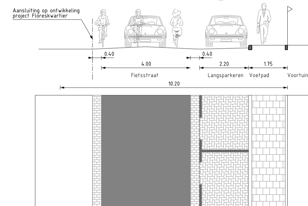
PROFIEL 57 SCHAAL 1 : 100 VO-03 Floreslaan
