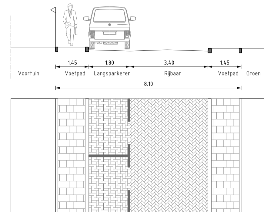
PROFIEL 54 SCHAAL 1 : 100 VO-03 Timorstraat
