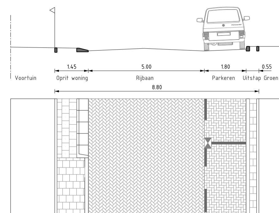
PROFIEL 49 SCHAAL 1 : 100 VO-03 Surinamesingel (zuid)
