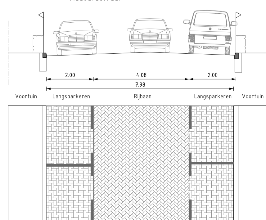
PROFIEL 60 SCHAAL 1 : 100 VO-03 Madoerastraat
