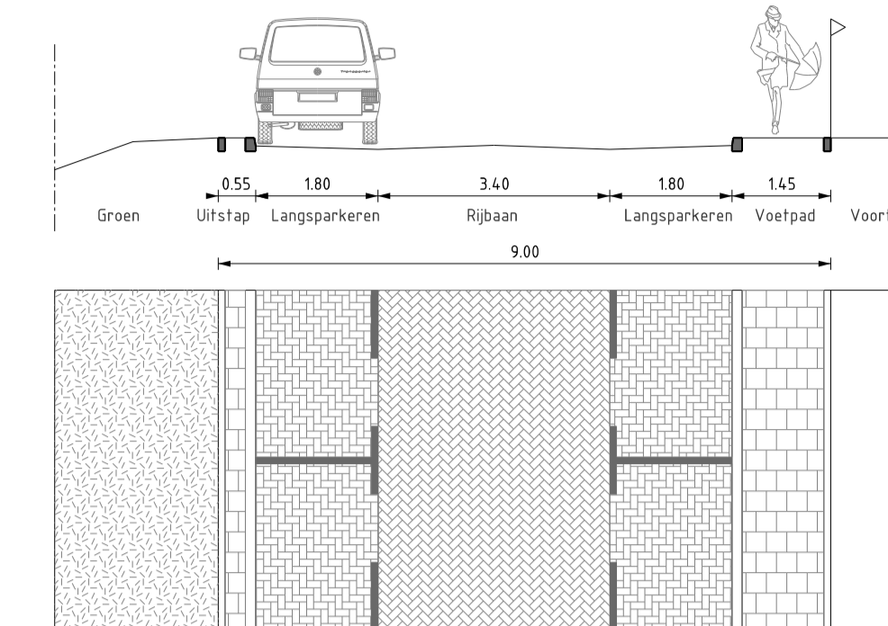
PROFIEL 50 SCHAAL 1 : 100 VO-03 Surinamesingel (noord)
