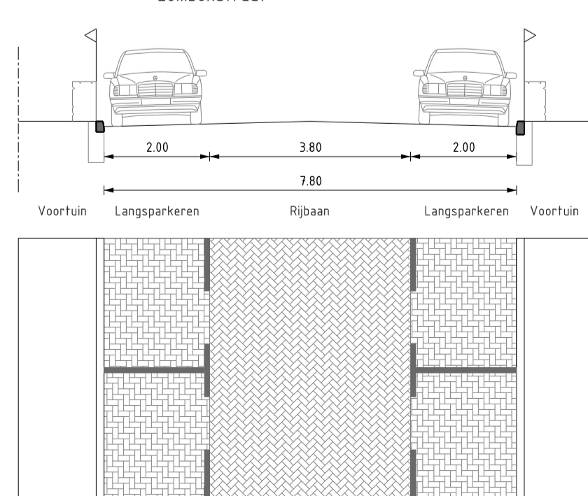
PROFIEL 61 SCHAAL 1 : 100 VO-03 Lombokstraat
