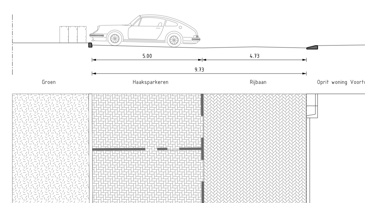
PROFIEL 58 SCHAAL 1 : 100 VO-03 Balistraat
