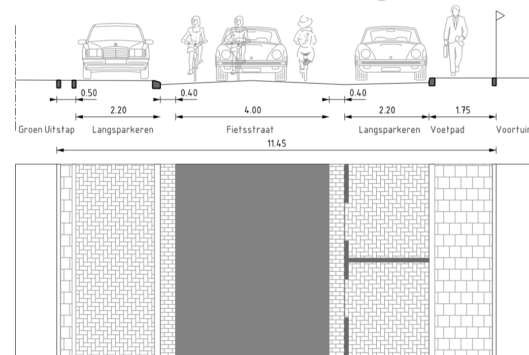
PROFIEL 56 SCHAAL 1 : 100 VO-03 Floreslaan
