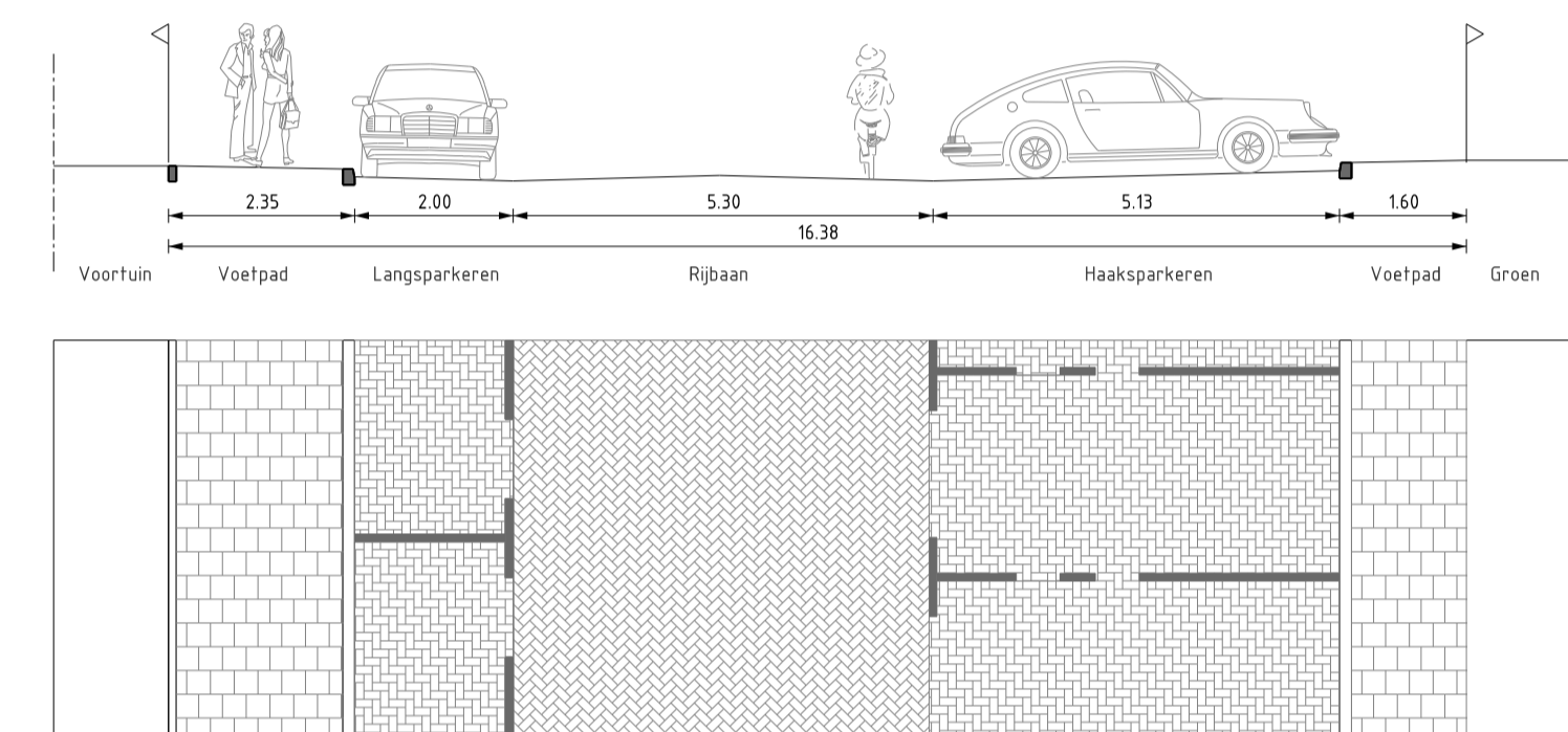
PROFIEL 52 SCHAAL 1 : 100 VO-03 Soendalaan
