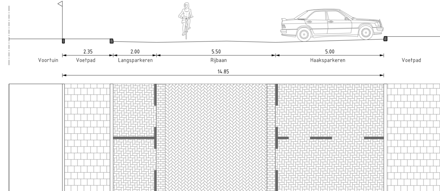
PROFIEL 34 SCHAAL 1 : 100 Soendalaan
