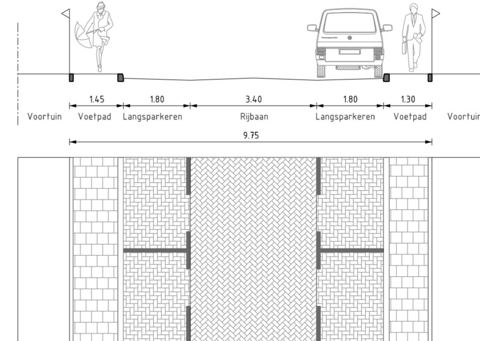
PROFIEL 40 SCHAAL 1 : 100 Sumatrasstraat
