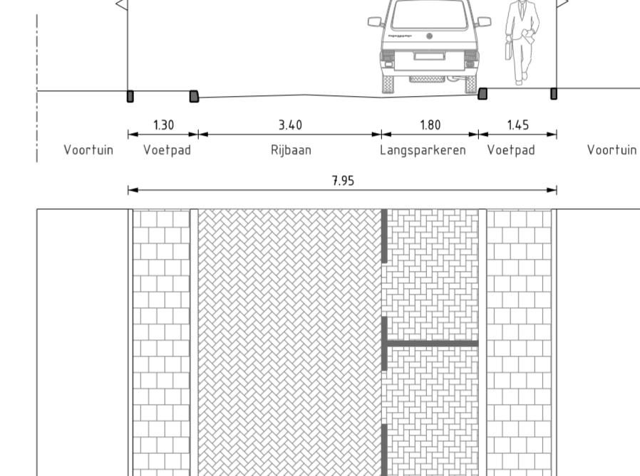
PROFIEL 36 SCHAAL 1 : 100 Javasstraat
