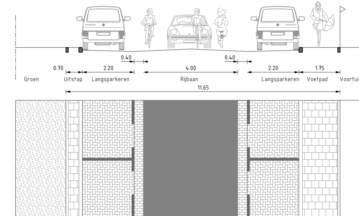
PROFIEL 46 SCHAAL 1 : 100 Curacaoaan (fietsstraat)
