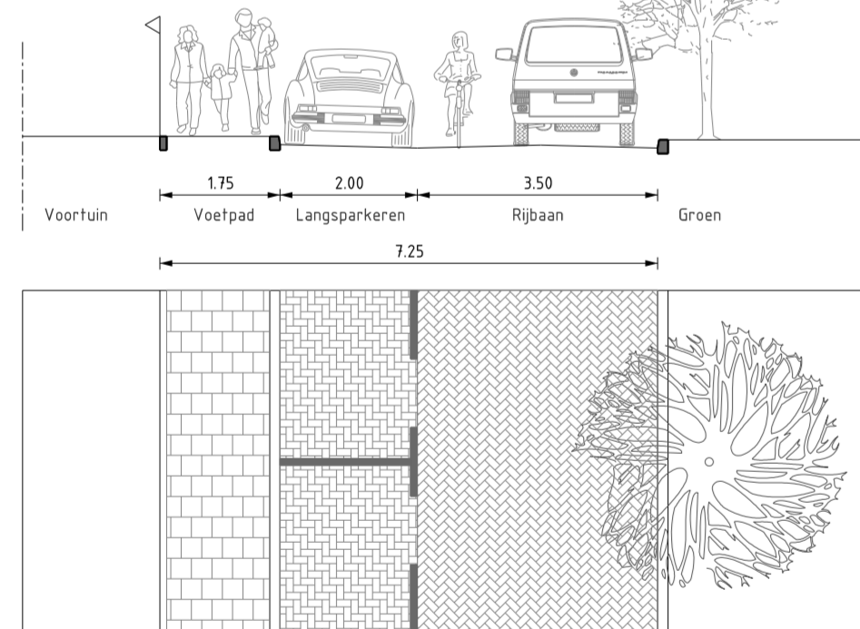
PROFIEL 37 SCHAAL 1 : 100 Burgemeester Pruisingsel
