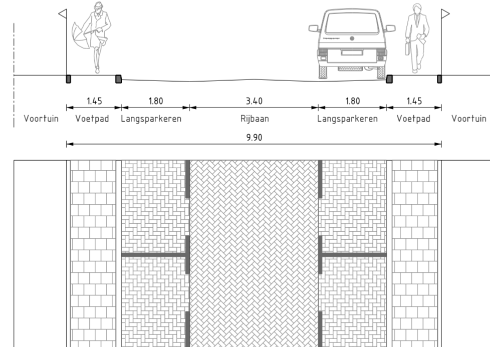
PROFIEL 39 SCHAAL 1 : 100 Celebesstraat
