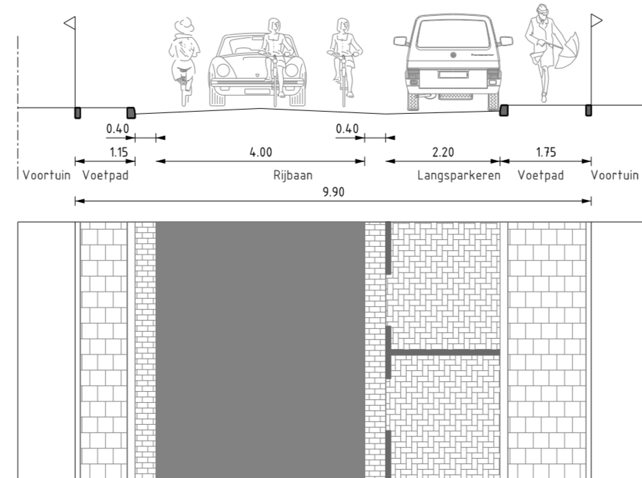
PROFIEL 45 SCHAAL 1 : 100 Curacaoaan (fietsstraat)
