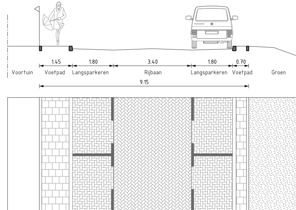
PROFIEL 42 SCHAAL 1 : 100 Surinamesingel (zuid)
