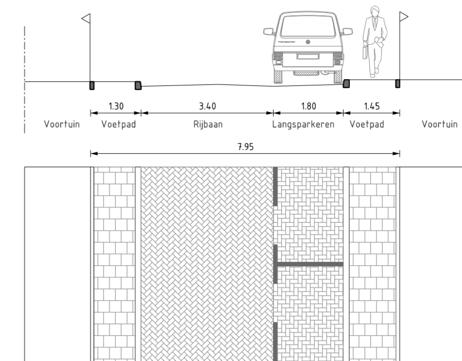
PROFIEL 32 SCHAAL 1 : 100 Boeroestraat
