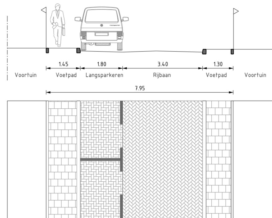
PROFIEL 29 SCHAAL 1 : 100 Bangkastraat
