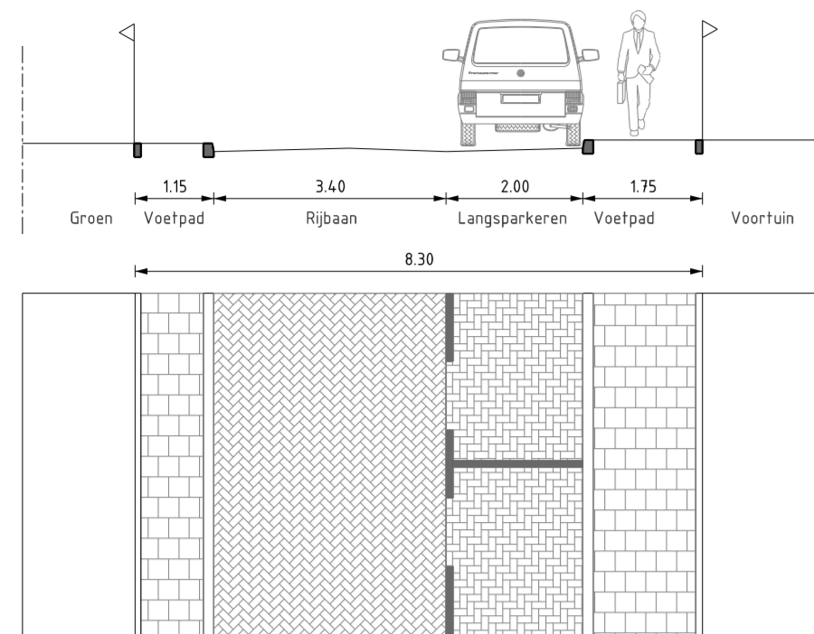
PROFIEL 28 SCHAAL 1 : 100 Insulindesingel
