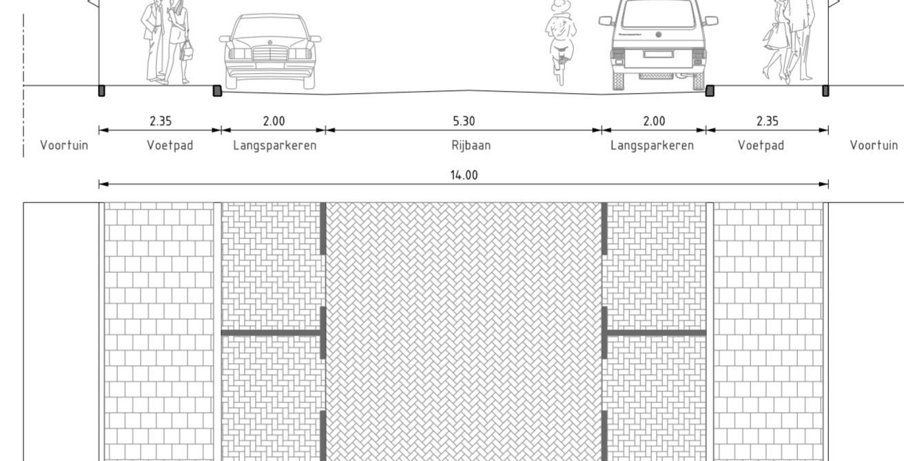
PROFIEL 35 SCHAAL 1 : 100 Soendalaan
