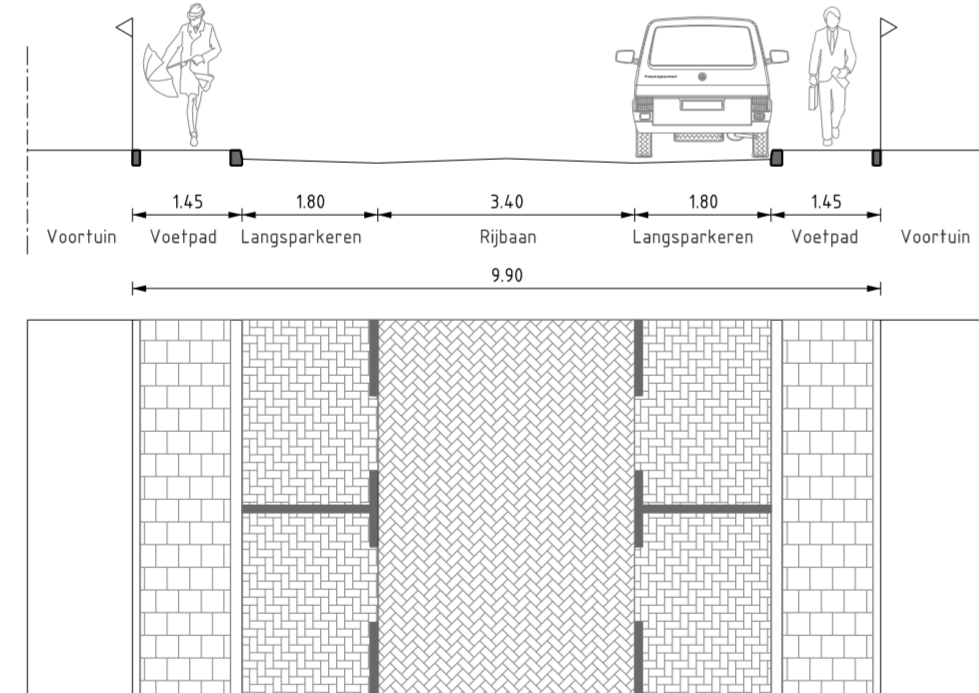
PROFIEL 38 SCHAAL 1 : 100 Borneostraat
