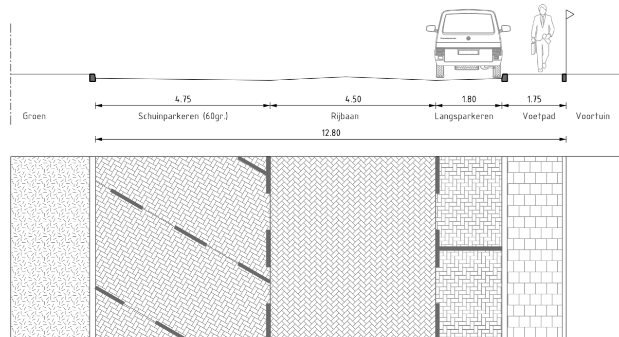
PROFIEL 43 SCHAAL 1 : 100 Insulindesingel
