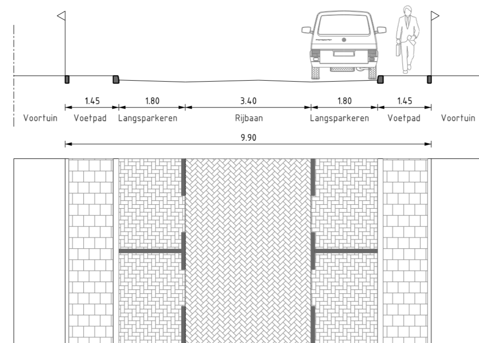
PROFIEL 30 SCHAAL 1 : 100 Molukkenstraat
