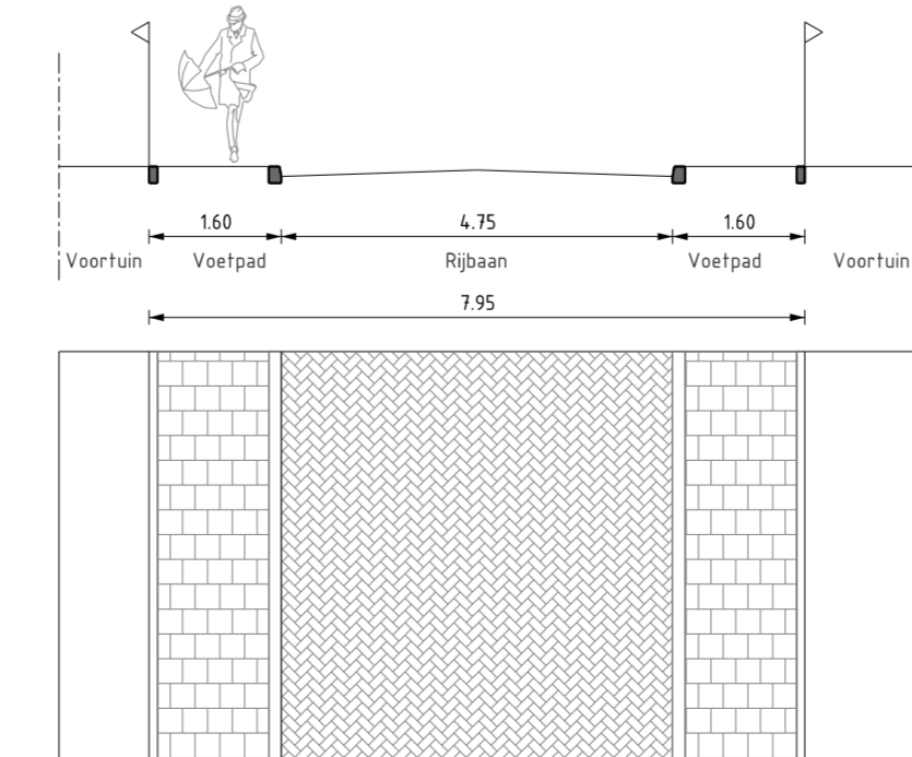
PROFIEL 44 SCHAAL 1 : 100 Arubastraat
