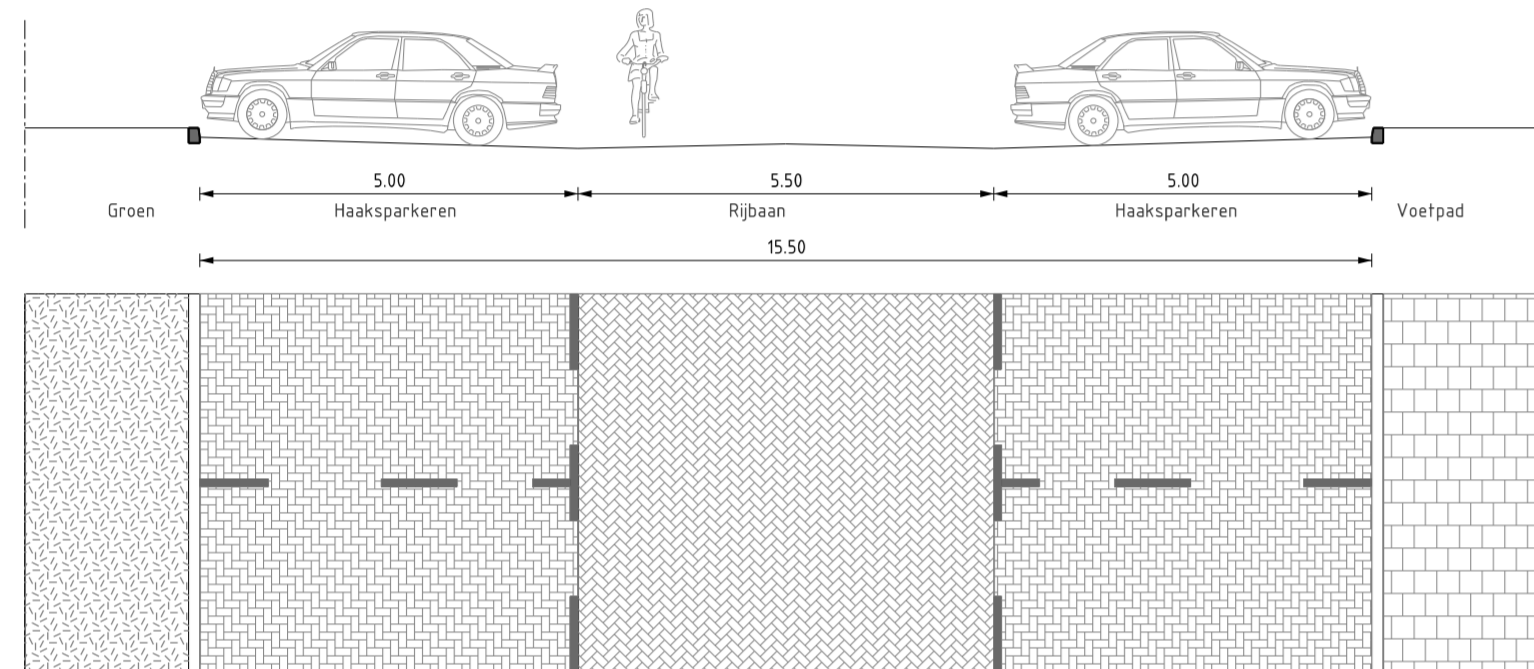
PROFIEL 33 SCHAAL 1 : 100 Borneostraat
