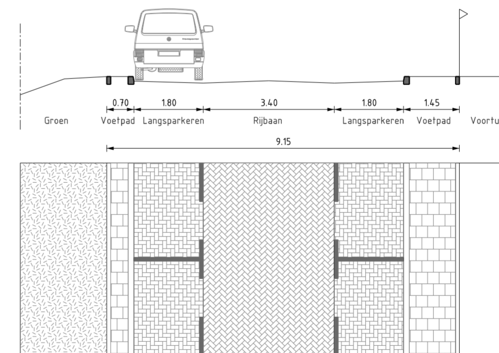
PROFIEL 41 SCHAAL 1 : 100 Surinamesingel (noord)
