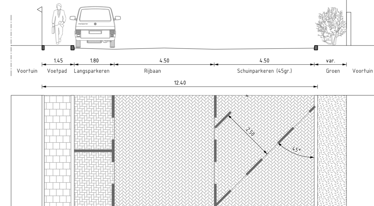
PROFIEL 31 SCHAAL 1 : 100 Borneostraat
